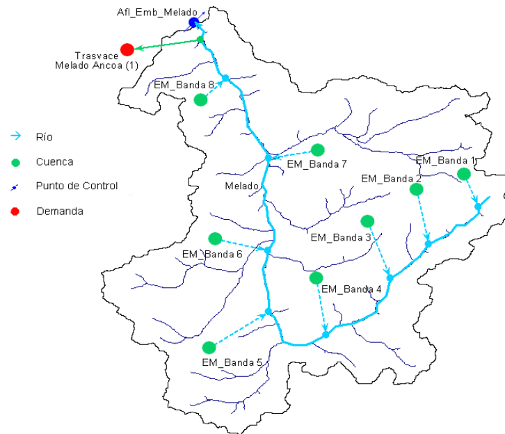
MAPA 9 ESQUEMA TOPOLÓGICO DE AFLUENTE A EMBALSE MELADO
