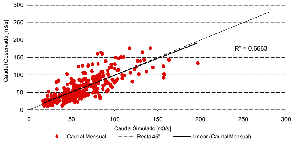
GRÁFICO 25 CORRELACIÓN DE CAUDALES MEDIOS MENSUALES DEL PERÍODO DE CALIBRACIÓN Y OBSERVADOS, AFLUENTE A LA LAGUNA LAJA (1966-1994)
